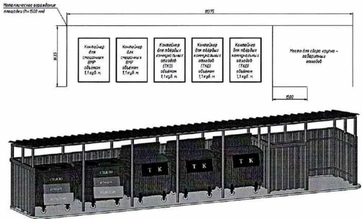
Рисунок 5.6 - Контейнерная площадка для сбора смешанных ВМР, ТКО и крупногабаритных отходов
