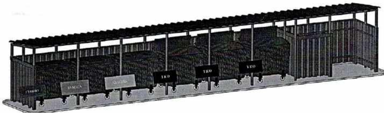
Рисунок 5.3 - Контейнерная площадка для сбора ВМР, ТКО и крупногабаритных отходов
