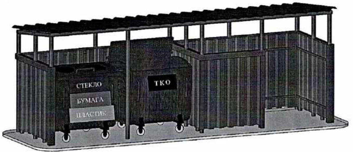
Рисунок 5.18- Контейнерная площадка для сбора смешанных ВМР, ТКО и крупногабаритных отходов
