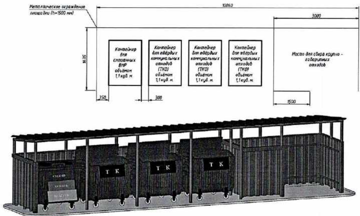
Рисунок 5.9 - Контейнерная площадка для сбора смешанных ВМР, ТКО и крупногабаритных отходов
